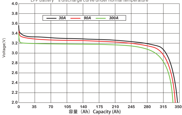
常温下 LFP类电池的放电特性曲线
